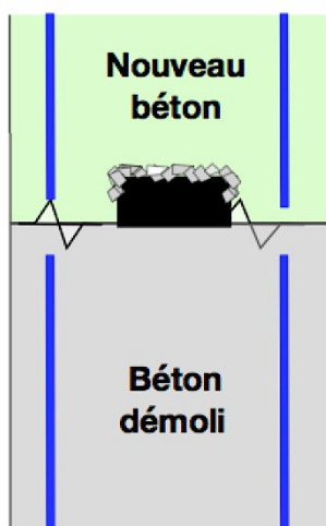
Coupe
